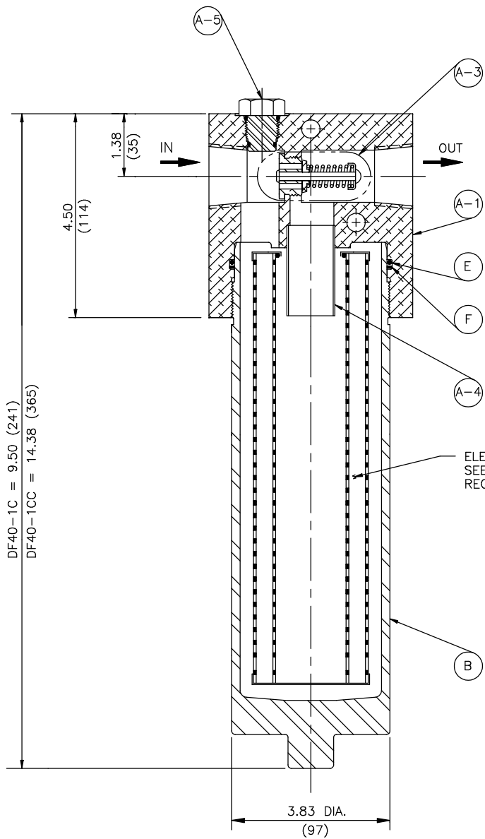
SECTION A-A
